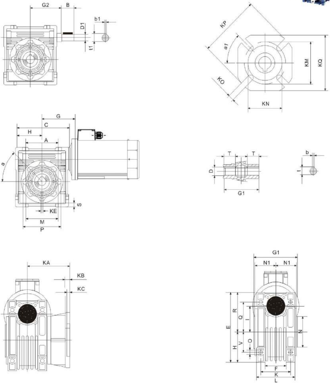
外型安装尺寸 Outline & installation size
