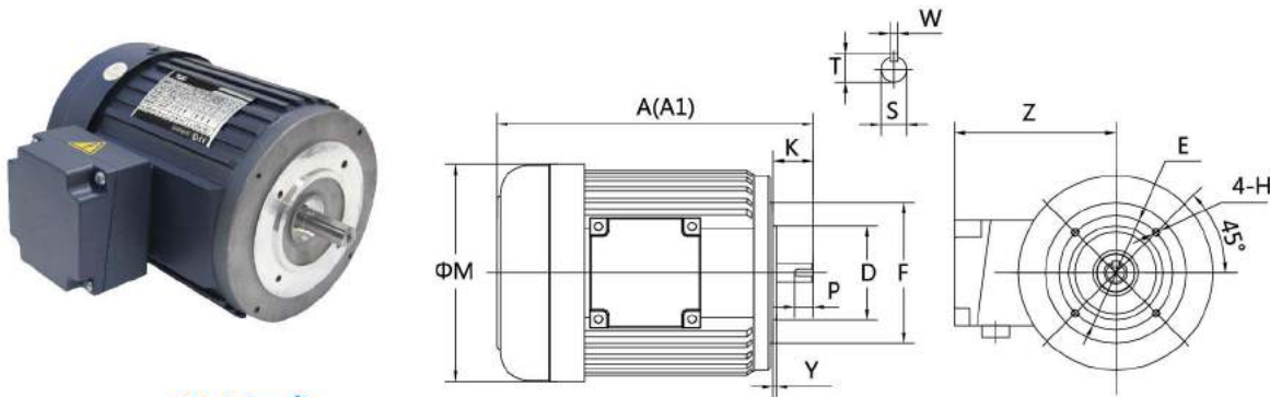
GV立式
