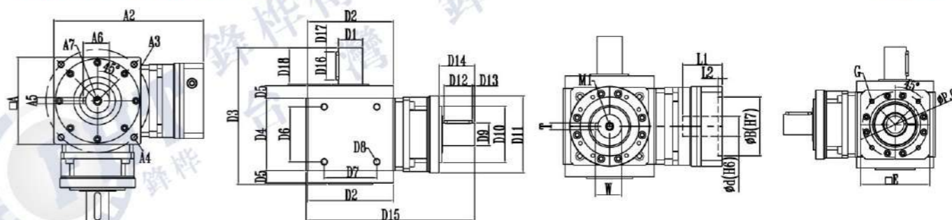
AATM080AS~~200BS-2AX-□-P-S□:尺寸表
