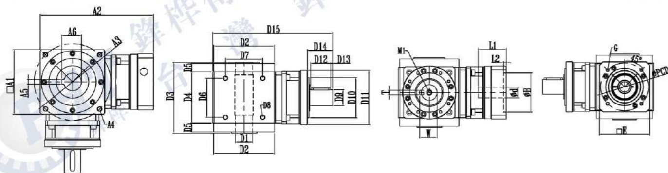
AATM080AS~~200BS-2AX-□-CR-S□:尺寸表
